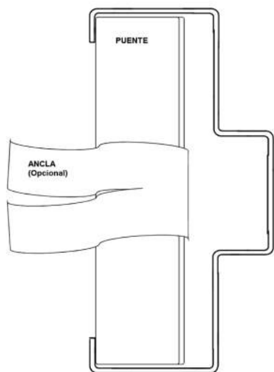
M.A.S. TIPO 4 AL CANTO DEL MURO
