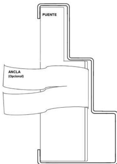
M.A.S. TIPO 6.1 AL CANTO DEL MURO
