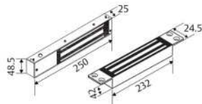
Electroimán 600LB
